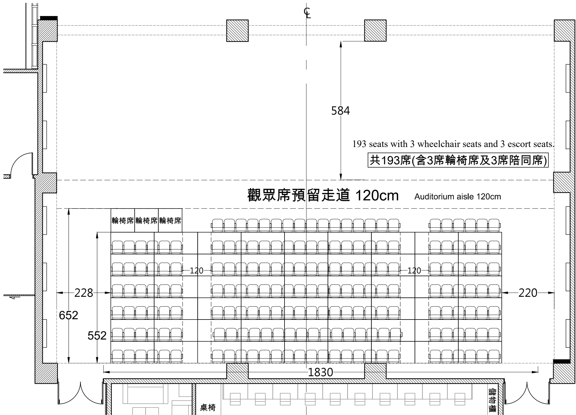
圖 (五) 多功能廳_觀眾席建議搭建位置Type B-直式 平面圖 (單位：公分)
